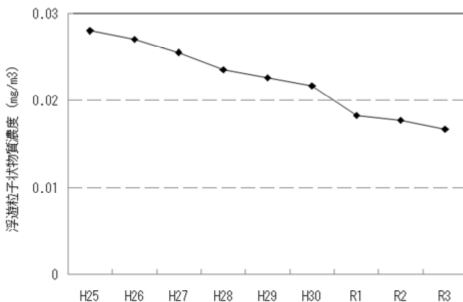
図 3-9 浮遊粒子状物質濃度の経年変化 (全局平均値)
