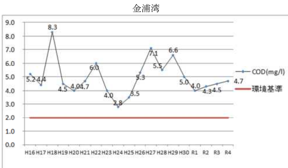
図 4-2 笠岡海域における COD (75%値) 経年変化
