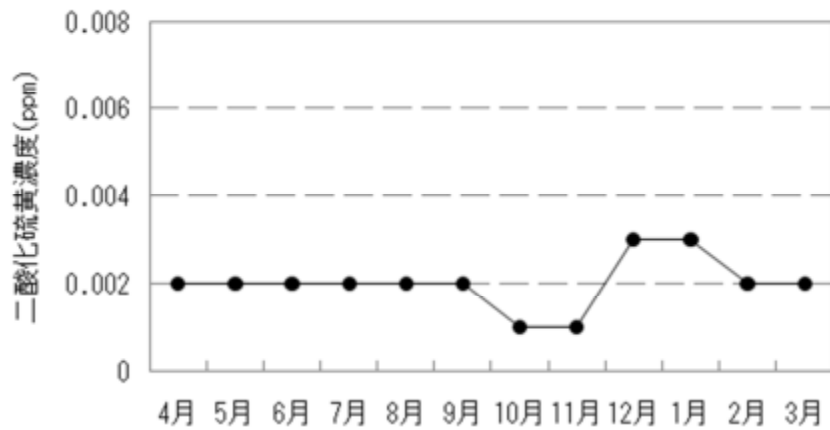
図3-2 寺間測定局における二酸化硫黄濃度の月別変化（令和4年度）
