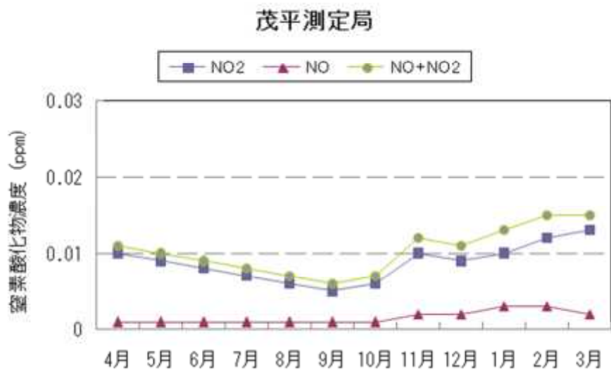
図 3-4 一般環境測定 2 局における窒素酸化物濃度の月別変化 (令和 4 年度)
