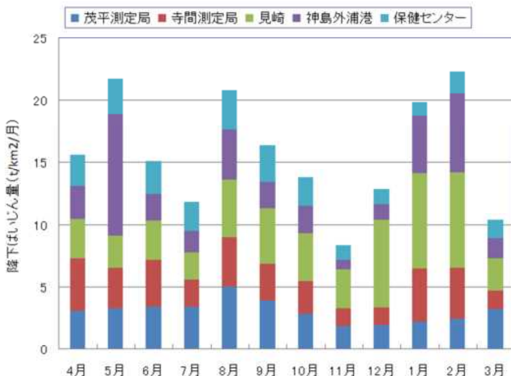
図3-12 降下ばいじん量の月別変化（令和4年度）
